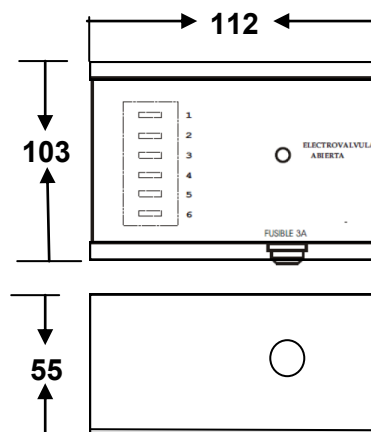
Fig 8 Dimensiones PQ 5001
