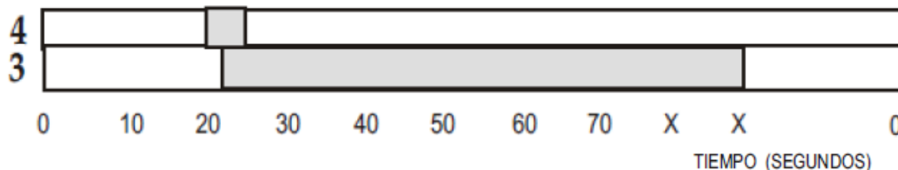
Fig 5 Diagrama de tiempos PQ 5001
