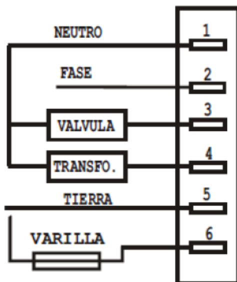
Fig 4 Diagrama de conexión PQ 5001
